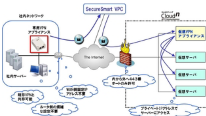
図 1. SecureSmart VPC システム構成概要
