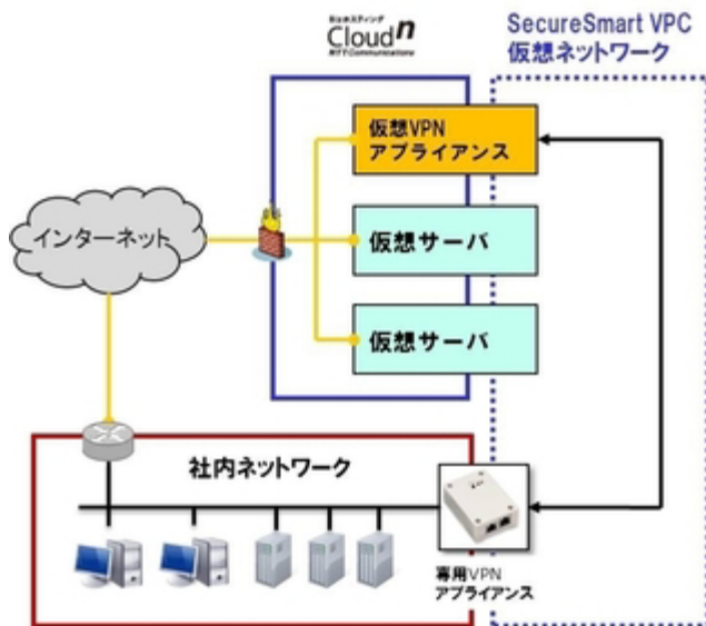
図 3. Cloud(n) (VLAN タイプ)
